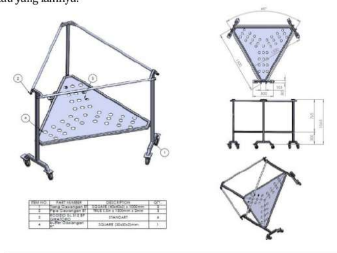
Gambar 3. Redesign Gawangan Dari Pipa
